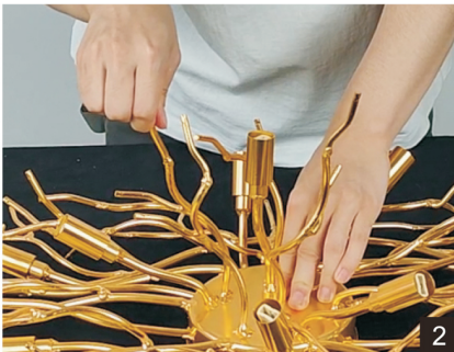
Schritt 2: Es wird empfohlen, die "Äste" vertikal in der Mitte zu platzieren, was den dreidimensionalen Sinn der Lampe verstärken kann.
