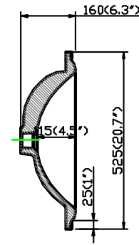
SECTION A-A
