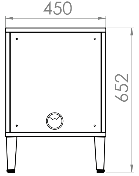
Rear view Arka görünüş
