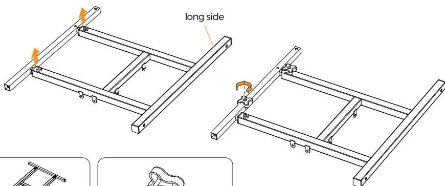
Left Leg
