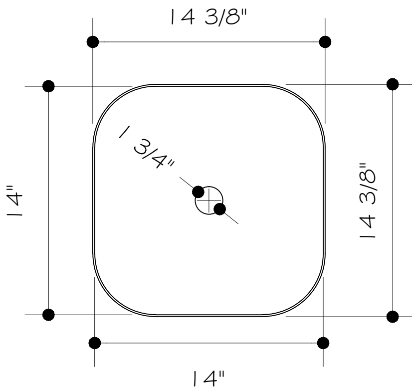
VISTA SUPERIOR
