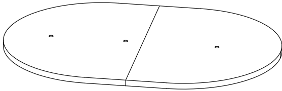
A -540x390mm(1pc)
