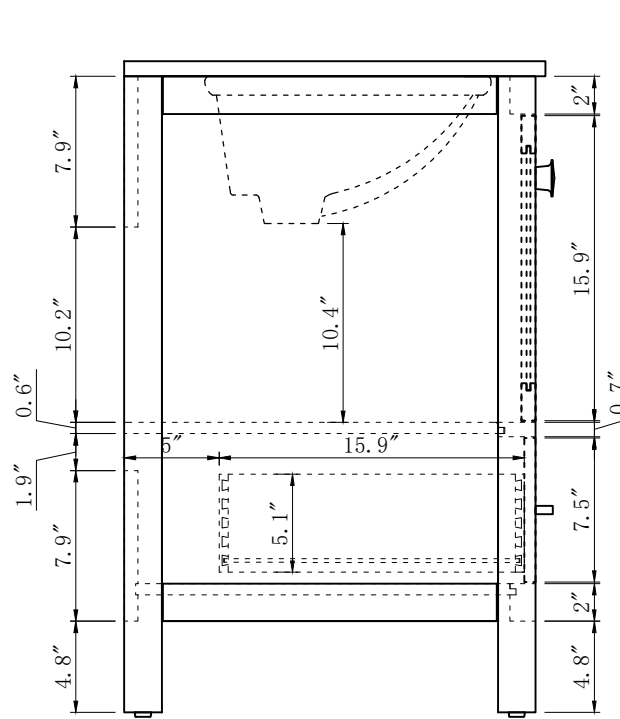
A-A SECTION
