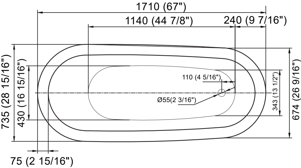
Top
