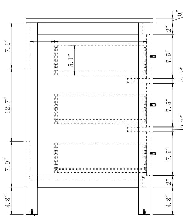
A-A SECTION
