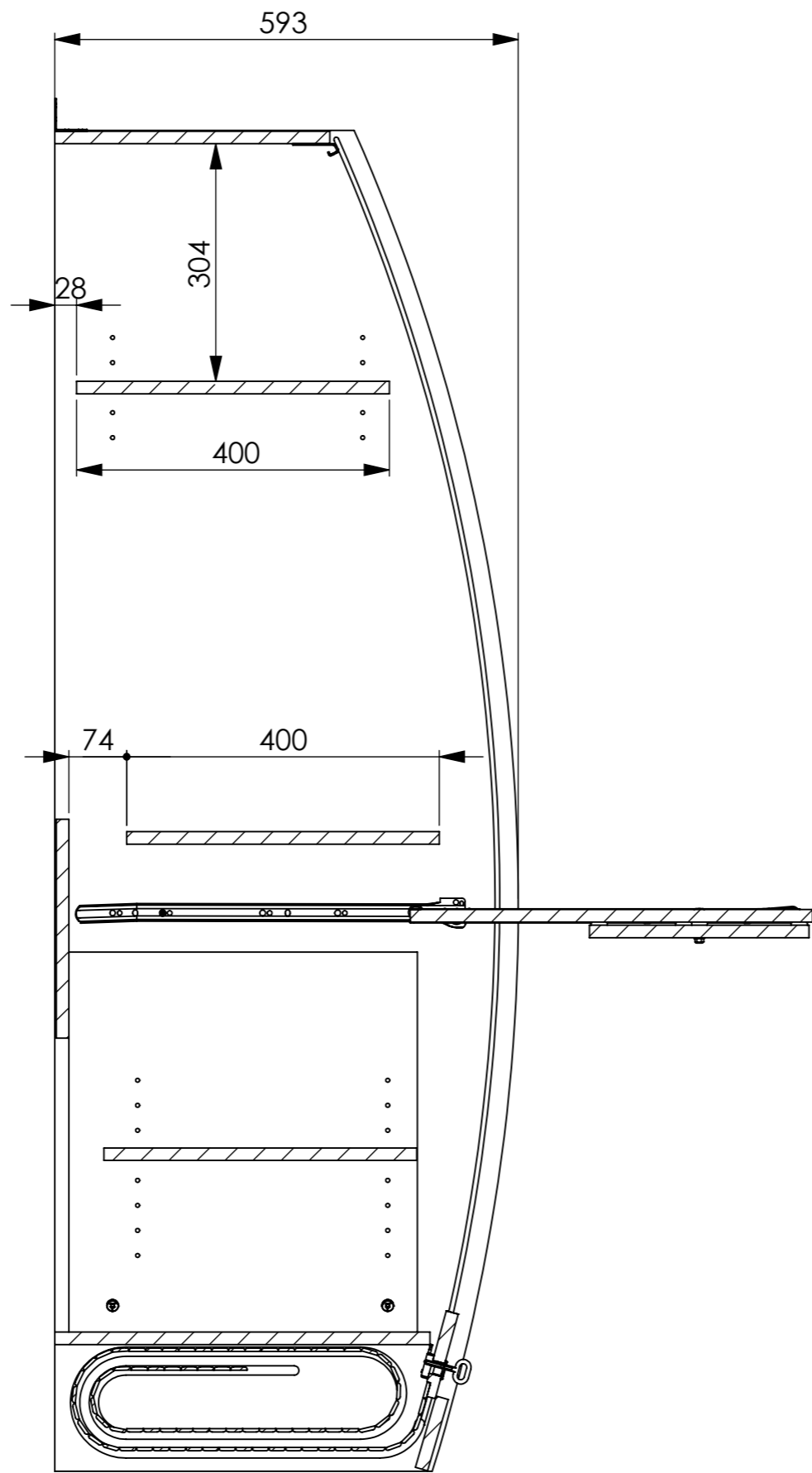
B-B (1 : 8)
