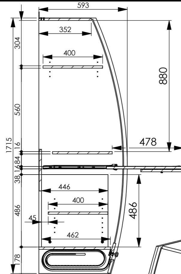
A-A (1 : 14.5)
