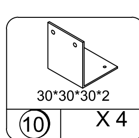
ANGLE BRACKET Escuadra TDK2007
