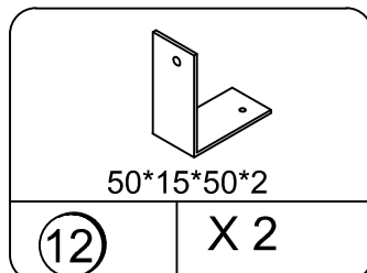
ANGLE BRACKET Escuadra TDK2010
