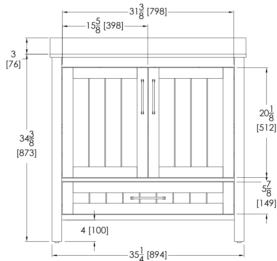
FRONT / DEVANT / FRENTE
