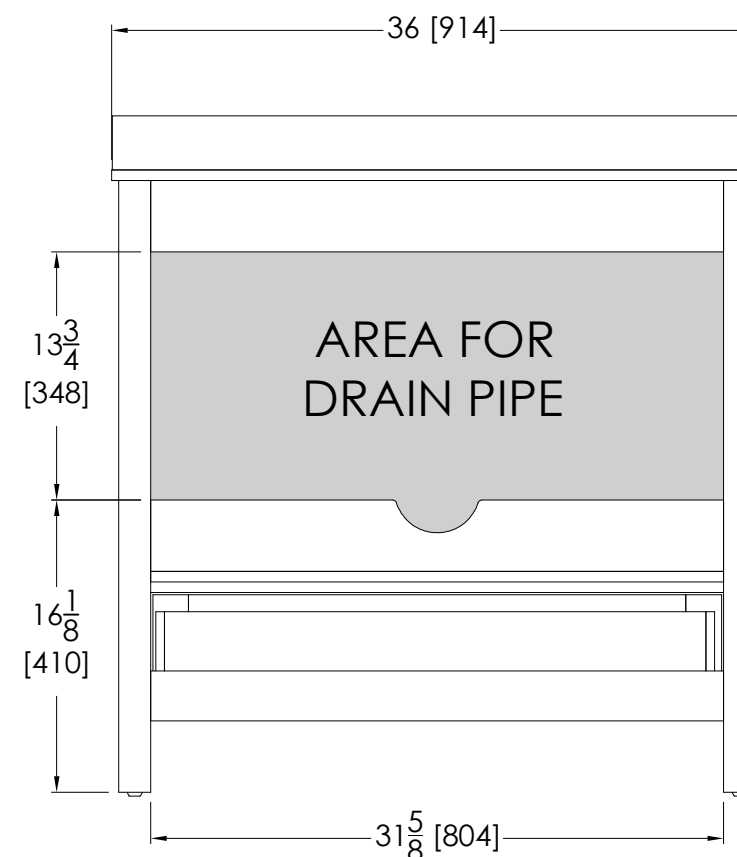
BACK / ARRIÈRE / ATRÁS
