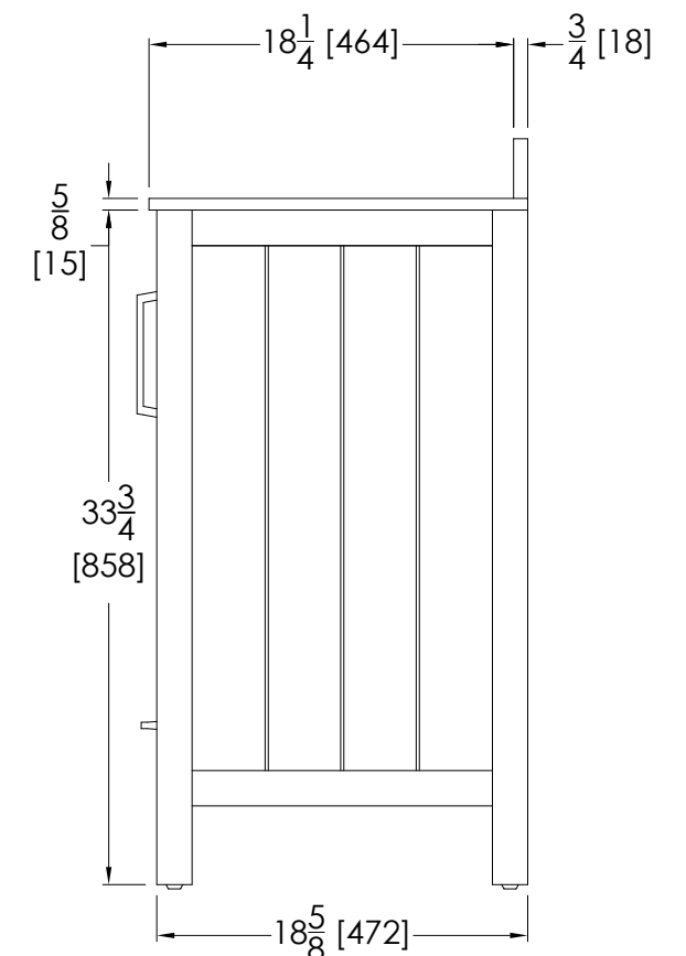
SIDE / CÔTÉ / LADO
