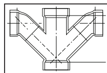
WYE de doble combinación/ curva de 1/8 SI
