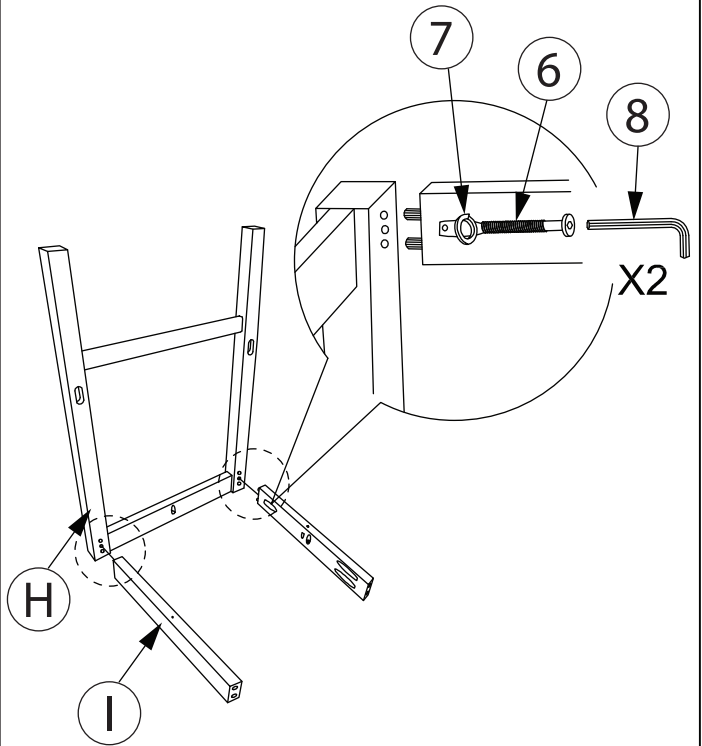
BARSTOOL: STEP 5
