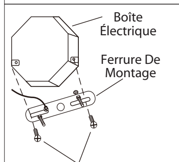
Vis De La Boîte Électrique (en sus)
