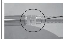
FIG. 11-3 Connecteur de la vanne attache au support de l'orifice sure le tuyau de brûleur. Détacher le connecteur de son support lors d'un changement d'orifice a un différent type de gaz.
