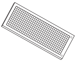
K 400*150*12mm(x1)
