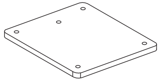
C 340*300*12mm(x1)
