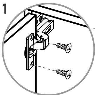
Ajuste de las bisagras Hinge adjustment
