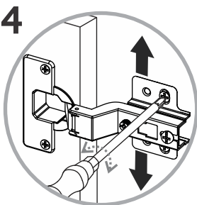
Ajuste de altura Height adjustment
