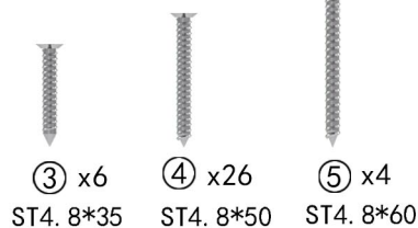
G. Jamb Screws
