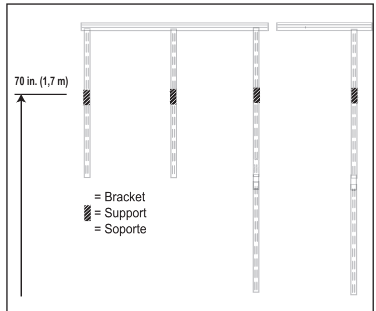
LONG HANG BRACKET LOCATION EXAMPLE EXEMPLE D'EMPLACEMENT DE SUPPORT DE SUSPENSION LONG EJEMPLO DE LA UBICACIÓN DEL SOPORTE PARA COLGADOR ALTO
