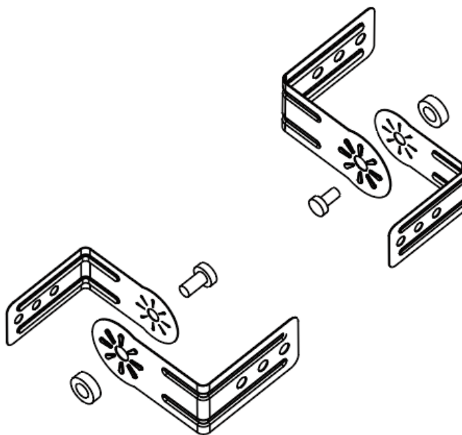
Tornillo M6 mm x 12 mm Cantidad: 2 piezas
