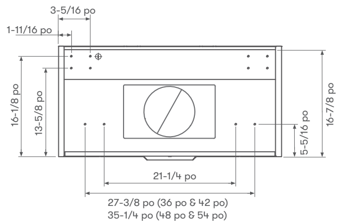
Vue arrière Dimensions de montage
