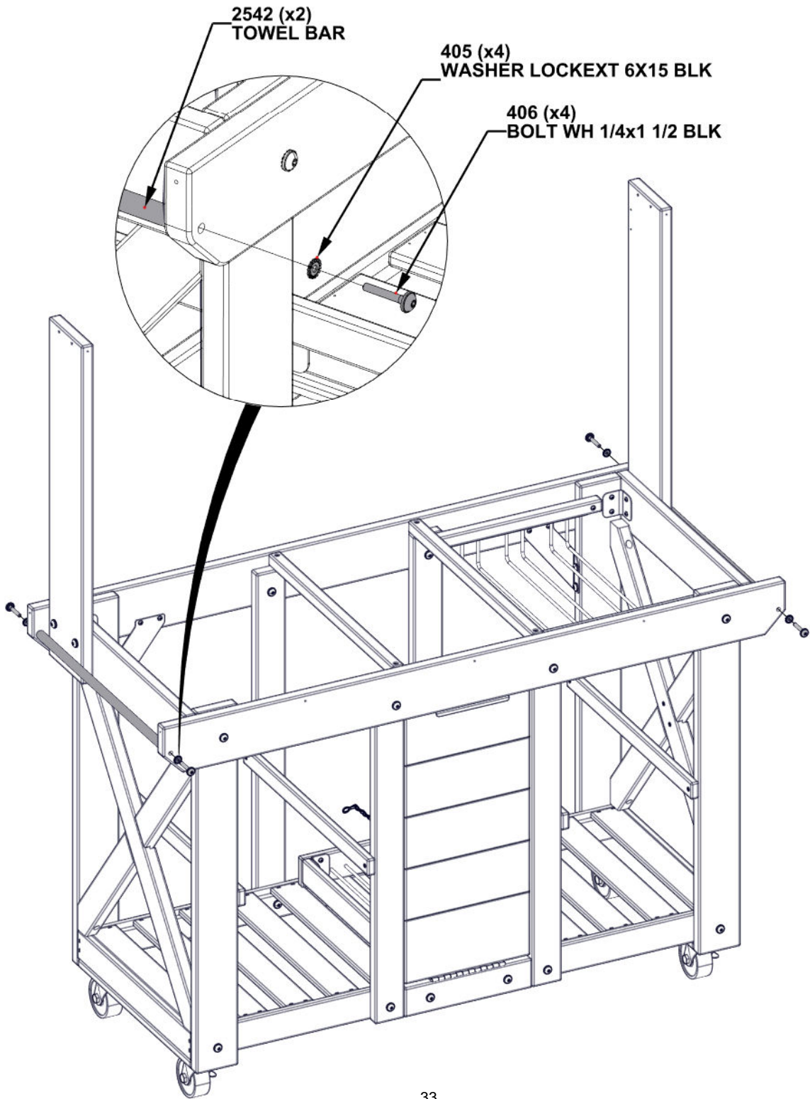
TOWEL BAR - A4M02542 (x2)
