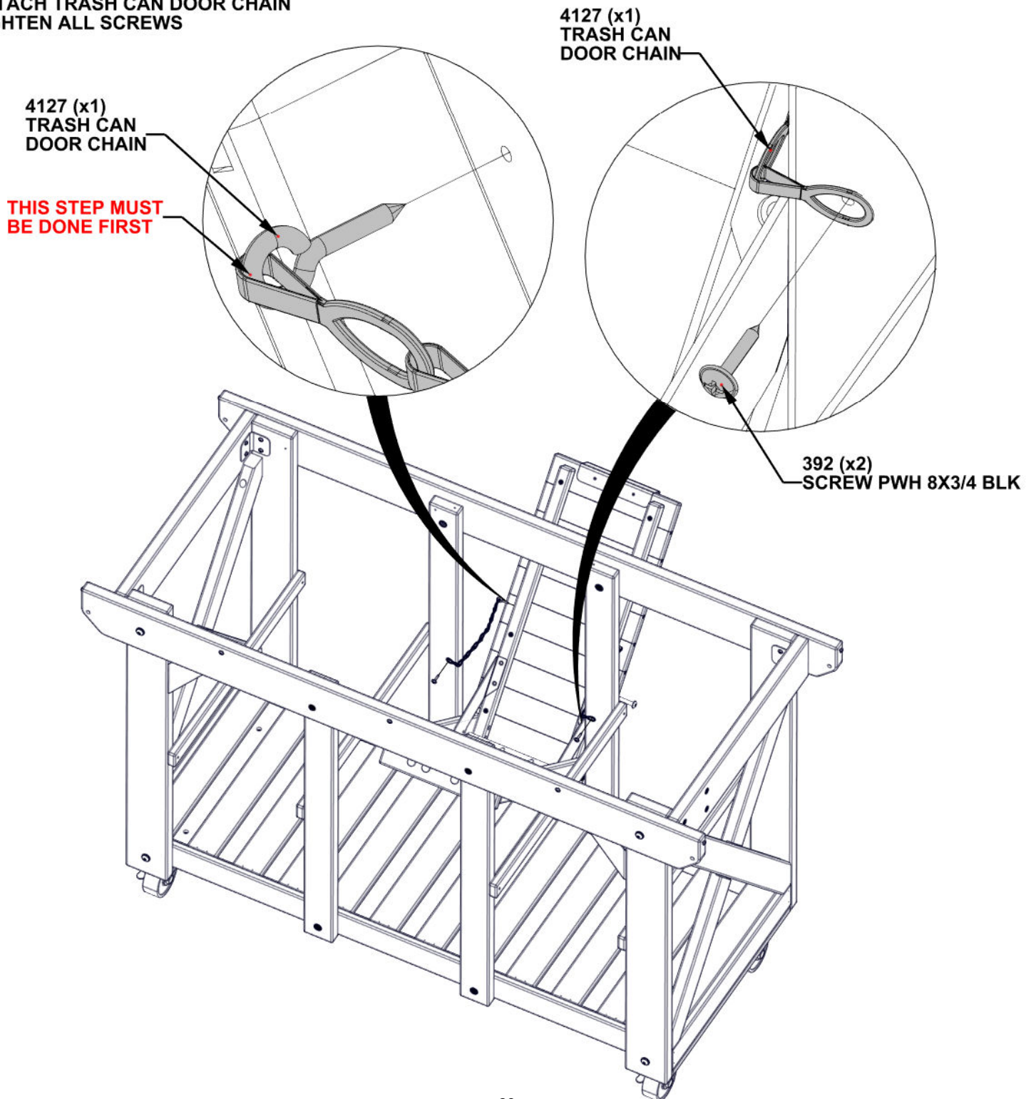
TRASH CAN DOOR CHAIN - A4M04127 (x2)
