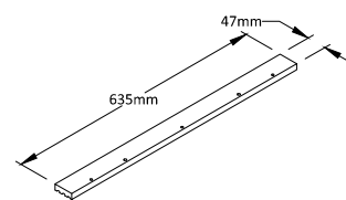
RAIL Qty:4
