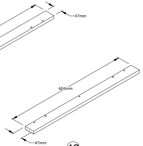
48 UPPER RAIL Qty:2
