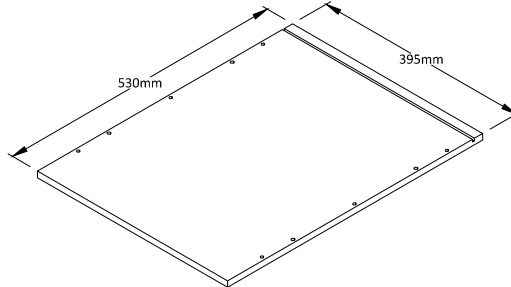
BOTTOM Qty:2
