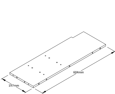
UPPER RIGHT PARTITION Qty:1
