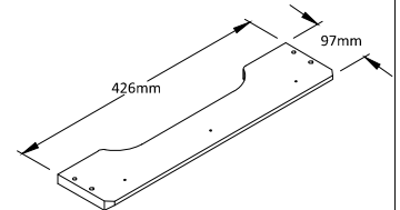
BOTTOM FRONT APRON Qty:2
