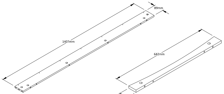
BACK RAIL Qty:2
