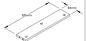
BOTTOM BACK APRON Qty:2
