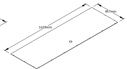
54 UPPER BACK PANEL Qty:1
