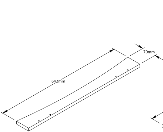
46 RAIL Qty:1
