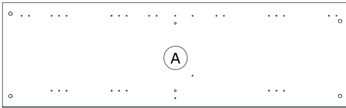
FI8629 1474x448x38mm
