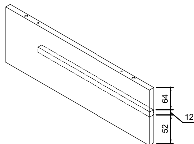
Left drawer divider Séparateur de tiroir gauche
