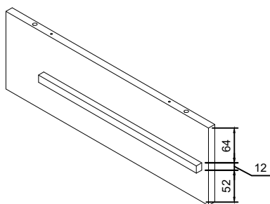
Right drawer divider Séparateur de tiroir droit
