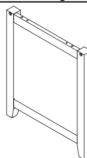
Lower left side frame Cadre latéral gauche inférieur
