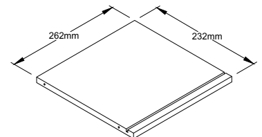
DRAWER BACK Qty:1
