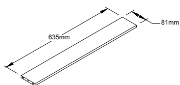
FRONT RAIL Qty:1
