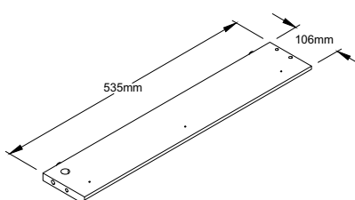
BOTTOM SIDE APRON, RIGHT Qty:2
