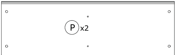
PI6507 1120x348x38mm
