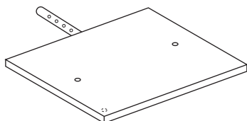
D 400*240*12mm(1pc)
