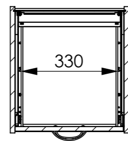
COUPE B-B ECHELLE 1 : 13
