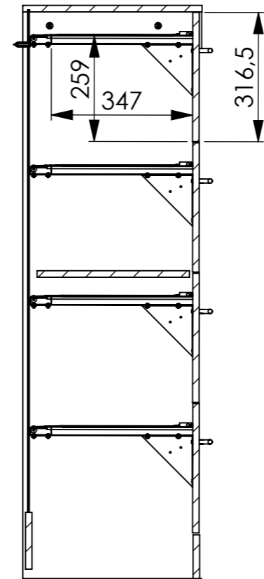
COUPE A-A ECHELLE 1 : 13
