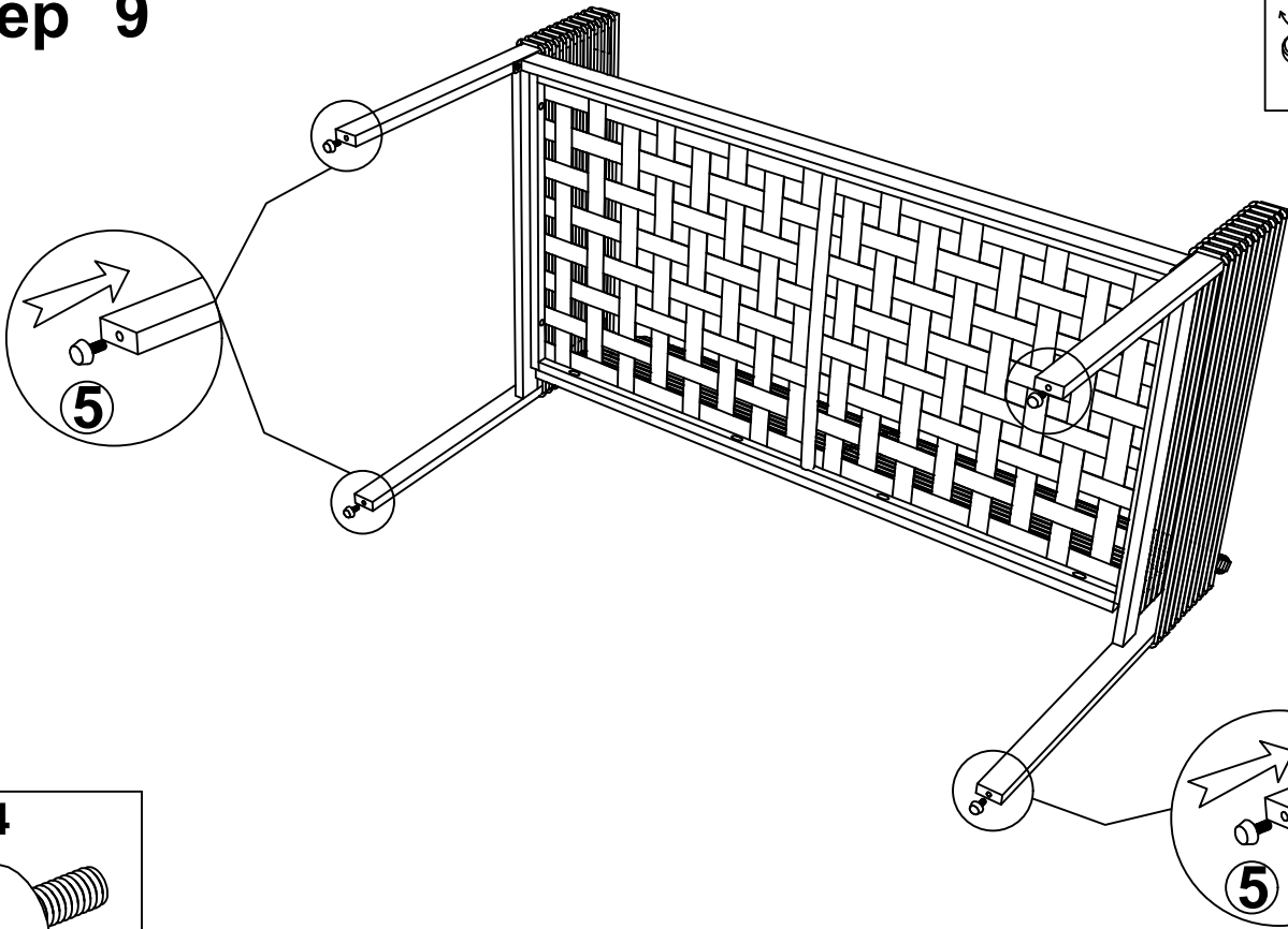
Leveler foot
