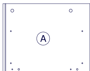
• FI7027 329x428x18mm
