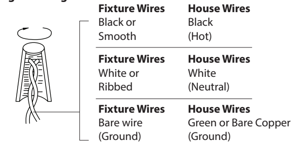
Fig. 3 Wiring
