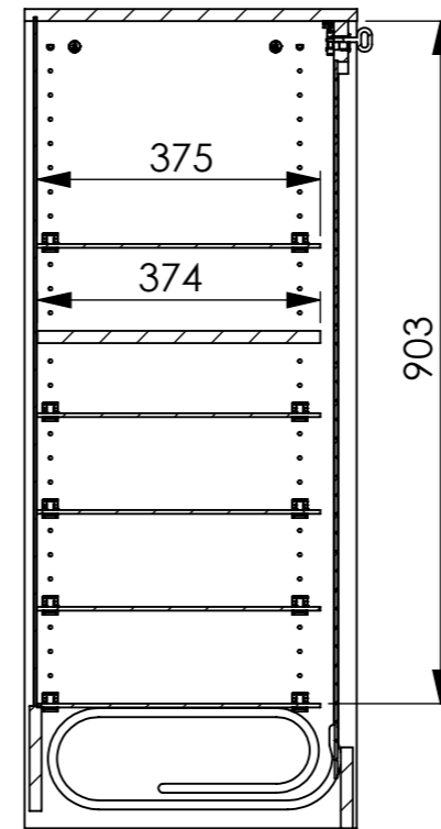
COUPE A-A ECHELLE 1 : 11
