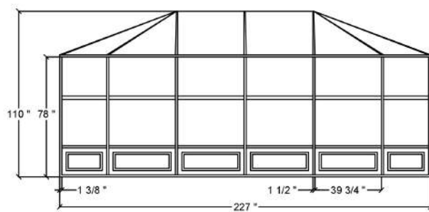
VUE DE CÔTÉ (LONGUEUR) SIDE VIEW (LENGTH)
