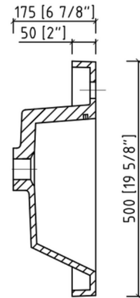
SECTION A-A
