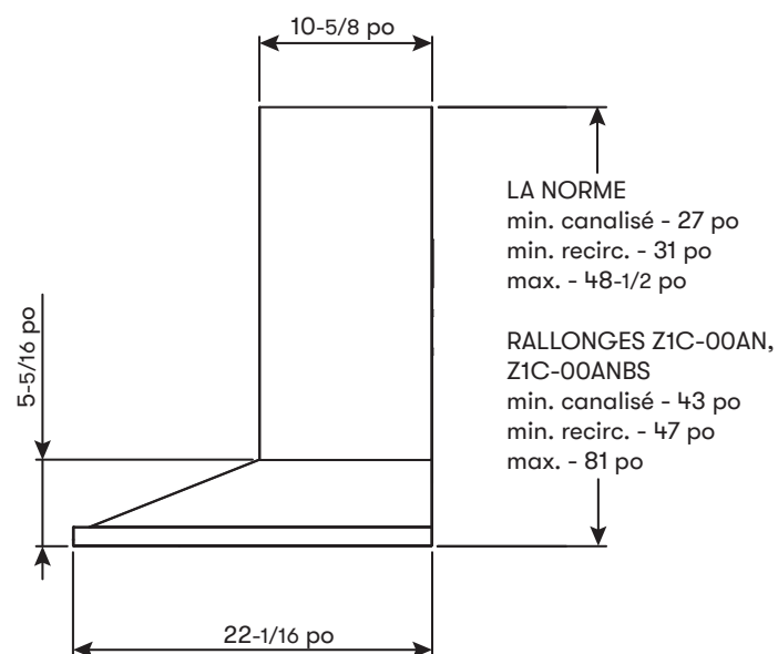
CÔTÉ
