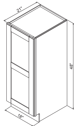
BT1821B 1 Door
