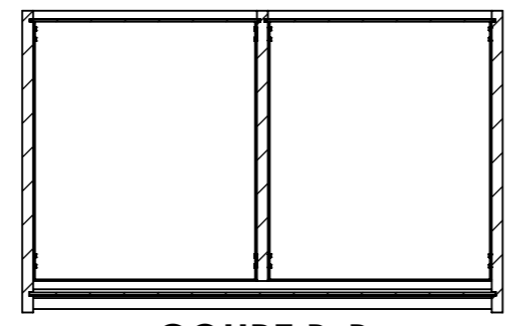
COUPE B-B ECHELLE 1 : 11
