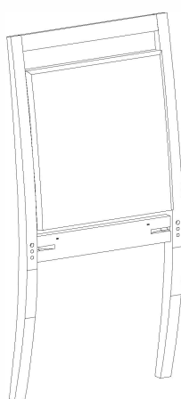
D1 (930x460x55mm) (36.61x18.61x2.16in)
