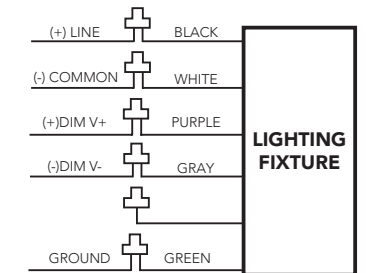
(0-10V Dimming Wiring Diagram)
