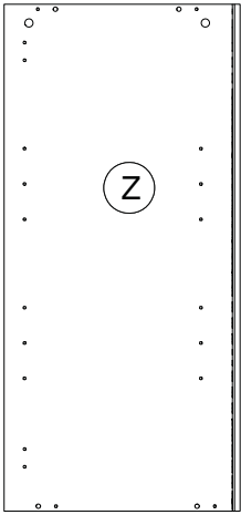
FI7868 918x428x18mm
