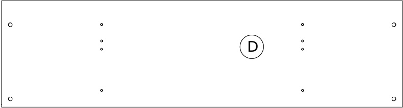
PI6748 1559x413x18mm
