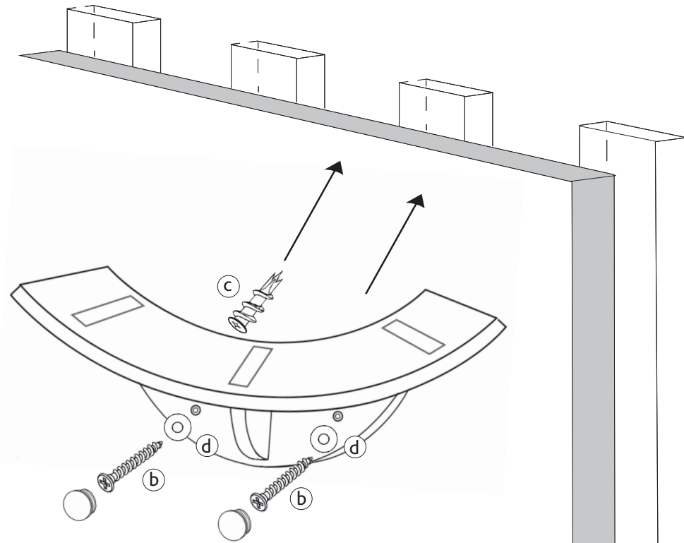
Wooden stud
