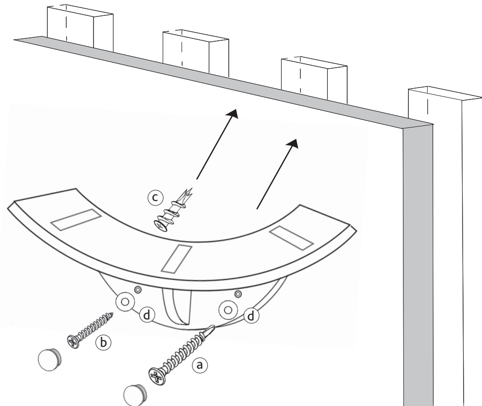
Metal stud
