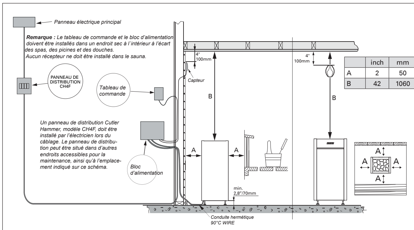
Figure 5. Commande du sauna / Distance de sécurité minimum / Installation du capteur
