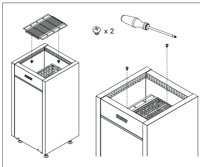
Figure 2. Installation de la grille de sécurité
