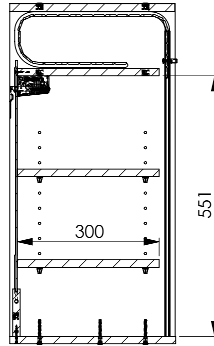
COUPE A-A ECHELLE 1 : 8
