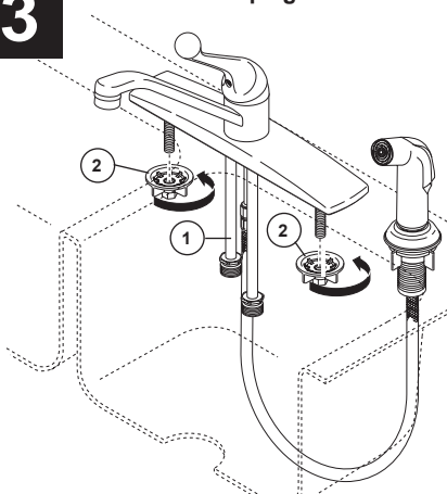
Monté sur plage
