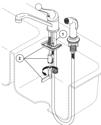
Monté dans un seul trou
