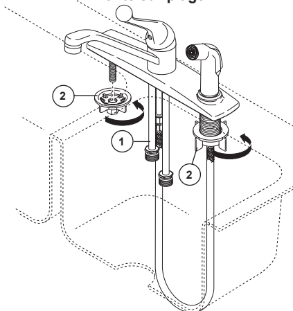
Monté sur plage
