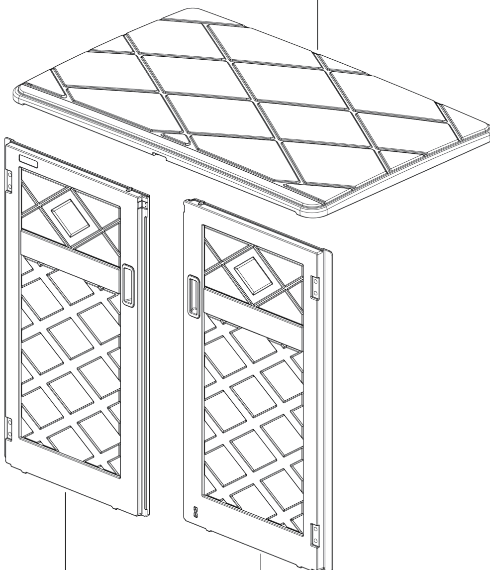
Left door BGS08006
