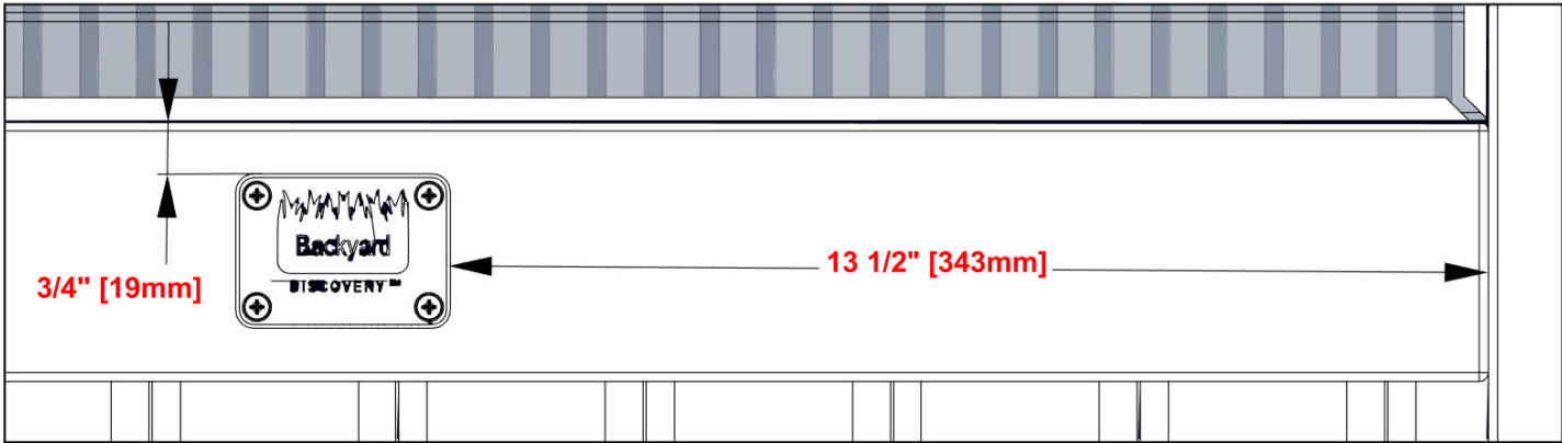
A4M02158 BYD ID TAG PATIO (x1)
