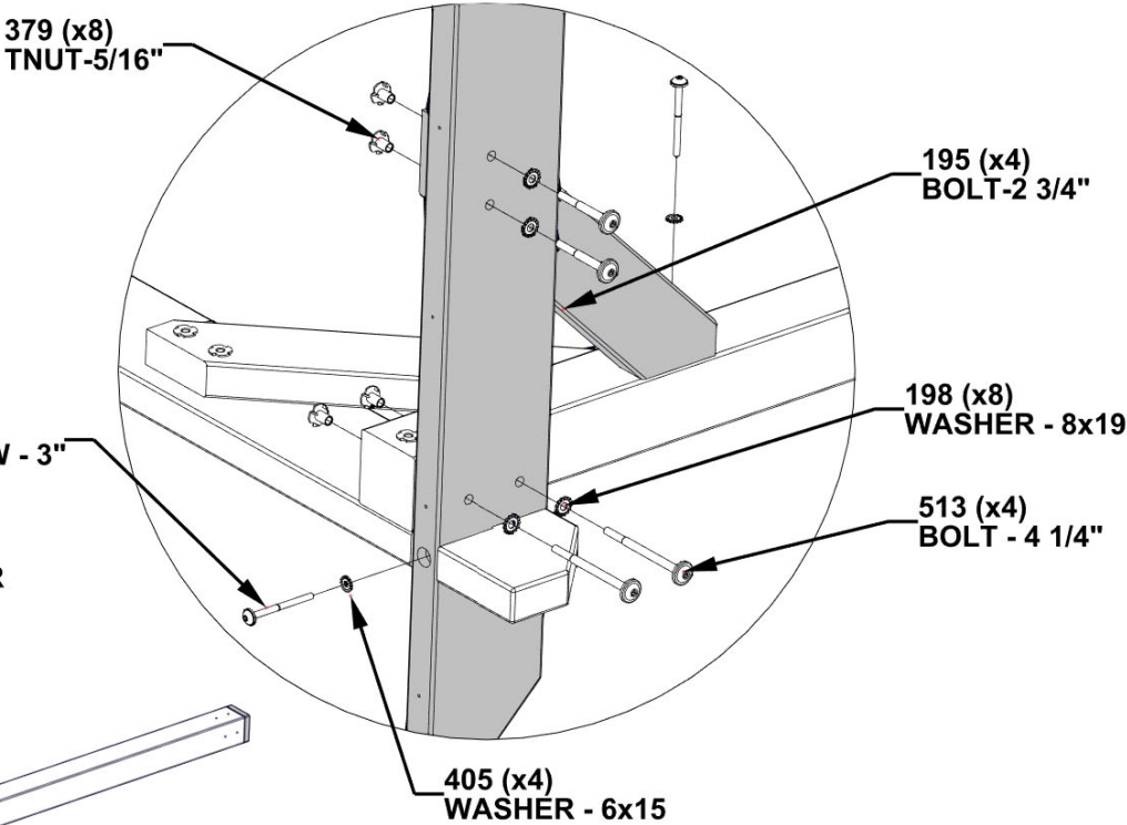
D07 (x2) PERGOLA RAFTER
