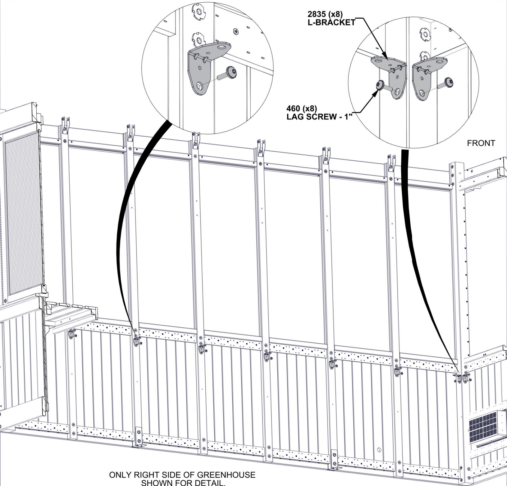
A4M02835 L-BRACKET (x8)
