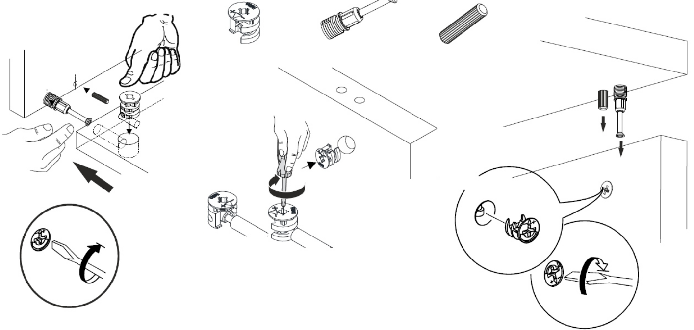
Minifix Gövde
