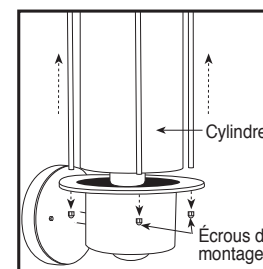
Figure 5 Appliques cylindriques
