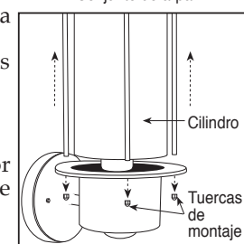
Figura 10 Unidades cilíndricas
